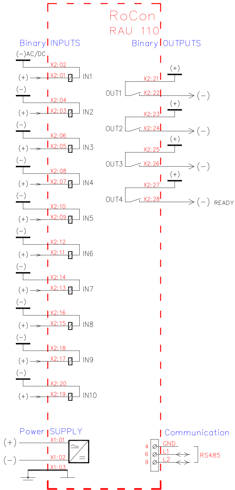
Фиг. 2b: Схема на външните връзки – RAU 110
