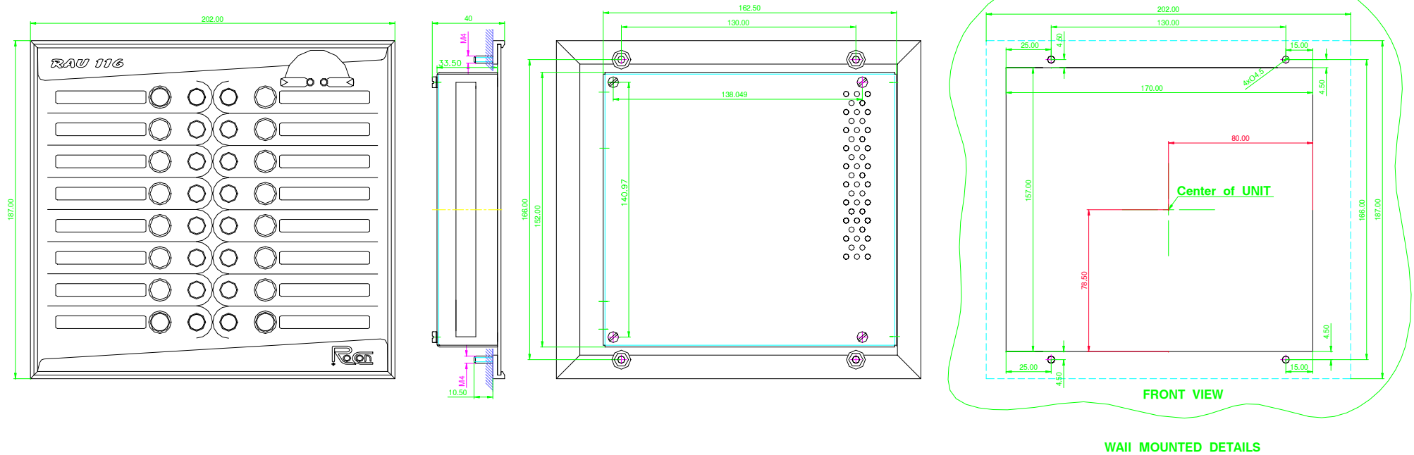
Фиг. 1: Габаритни и присъединителни размери (Схемата е валидна за RAU 116 и RAU 110)
