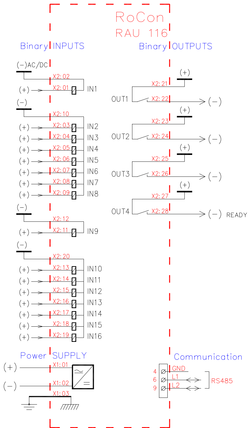
Фиг. 2а: Схема на външните връзки – RAU 116
